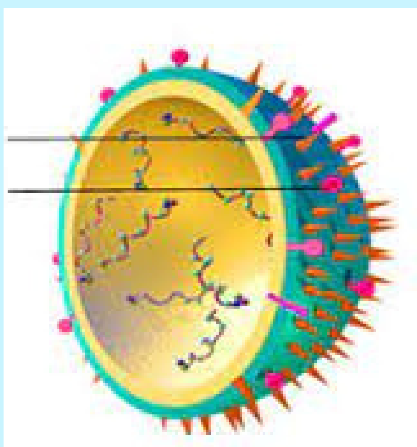
Slika 1. Model virusa
